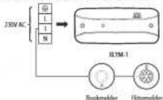
RLYM-1 – Bedrade ingangsaansluitingen
